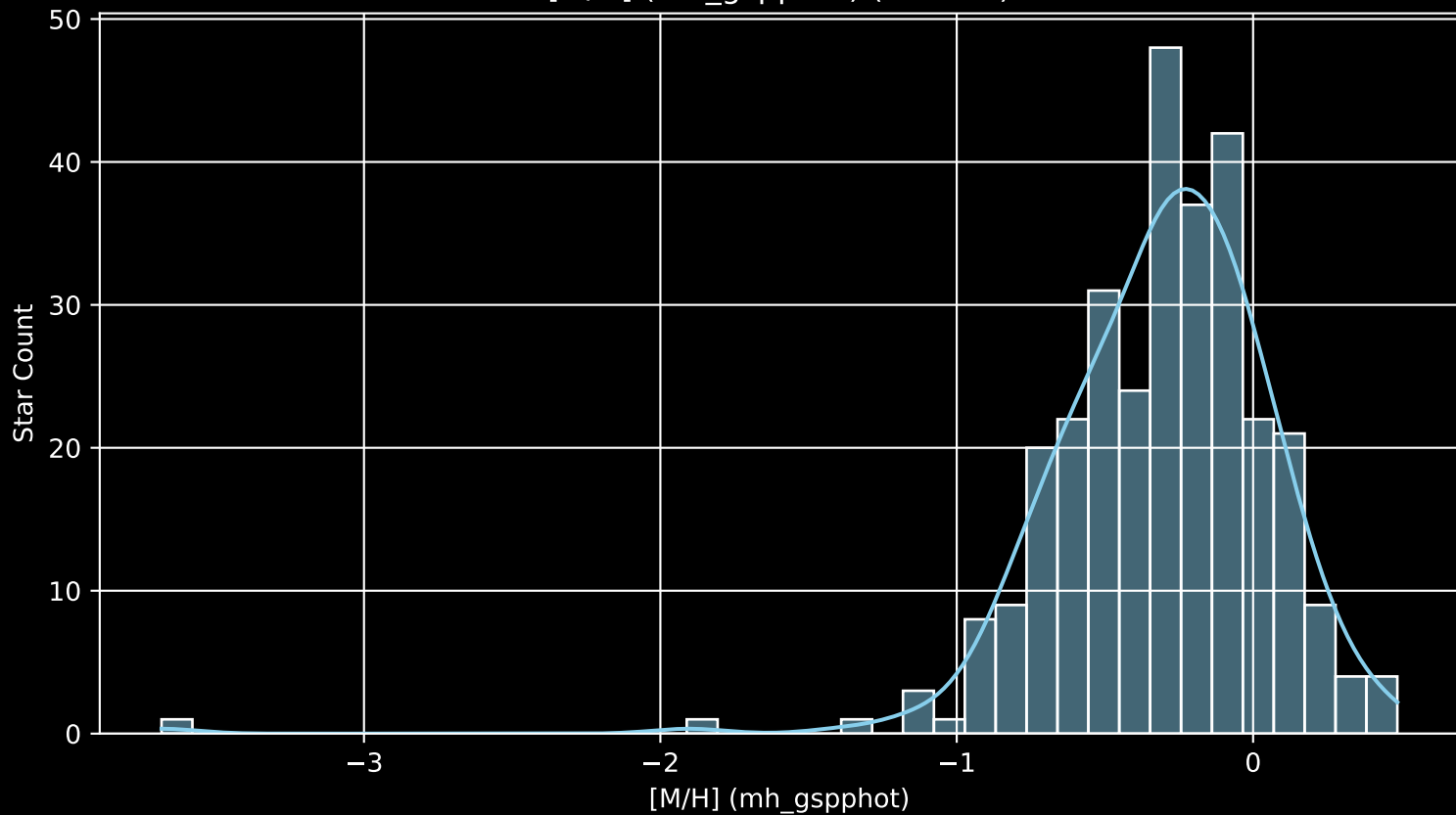
GALAH DR4 Field: [6959] [M/H] (mh_gspphot) (n= 308)
