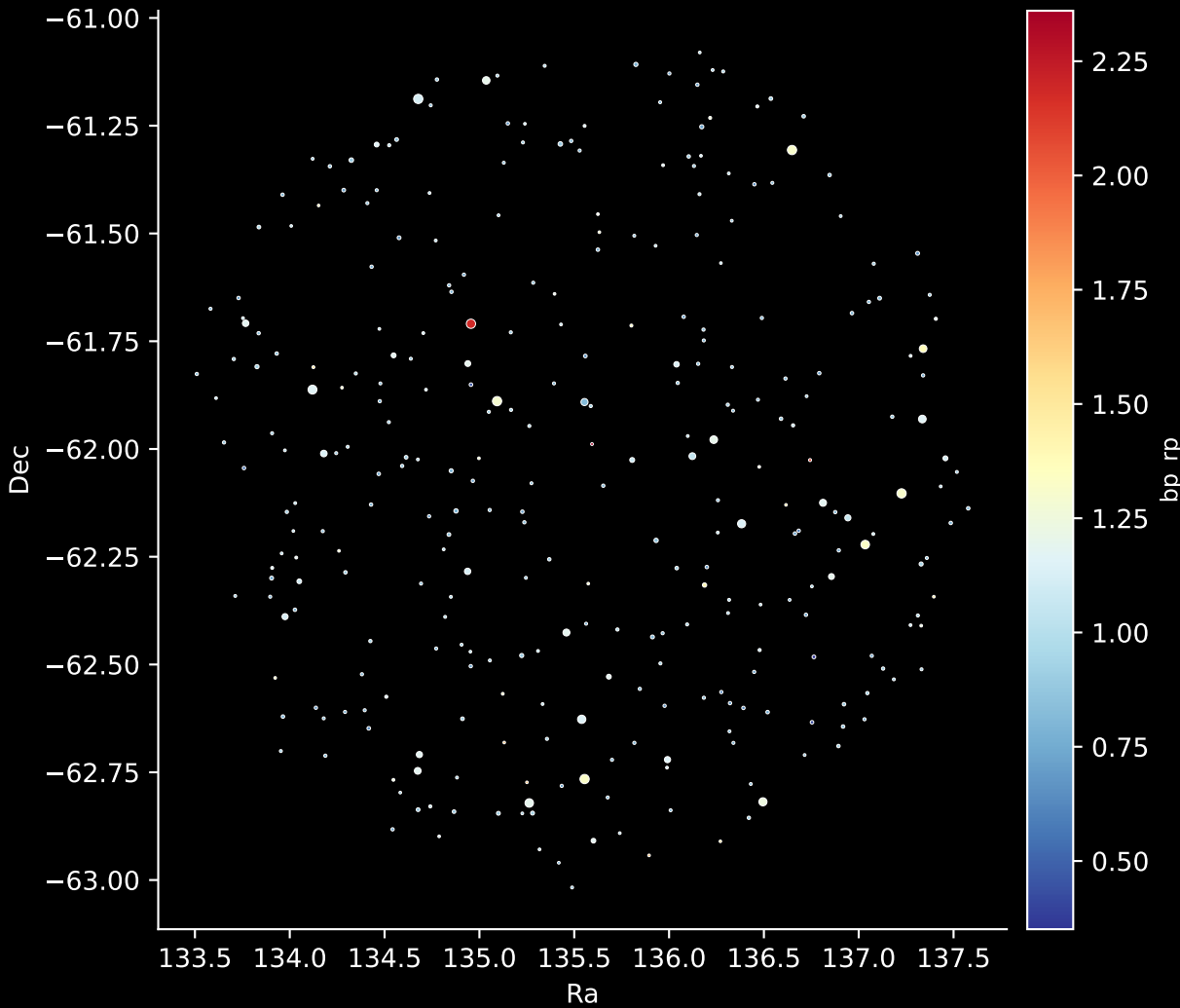
GALAH DR4 Field: [6959] Stars: 309
