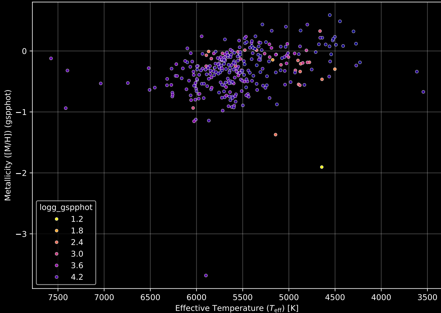
GALAH DR4 Field: [6959] Stellar Population Parameters (n= 309)
