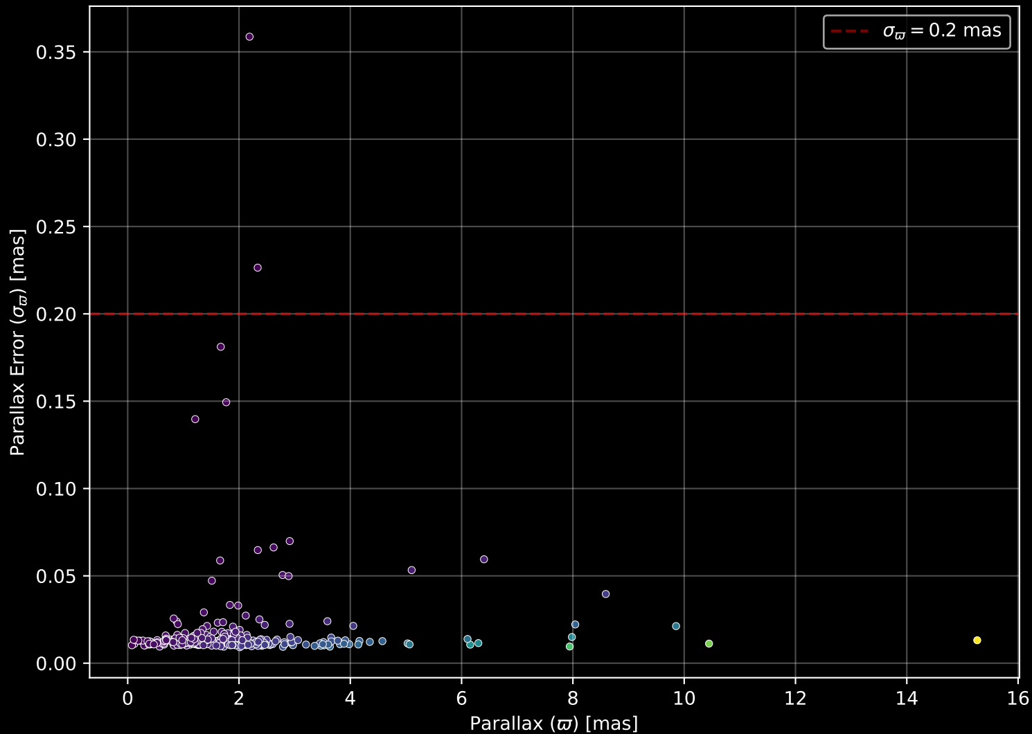
GALAH DR4 Field: [6959] Parallax Quality (n= 309)
